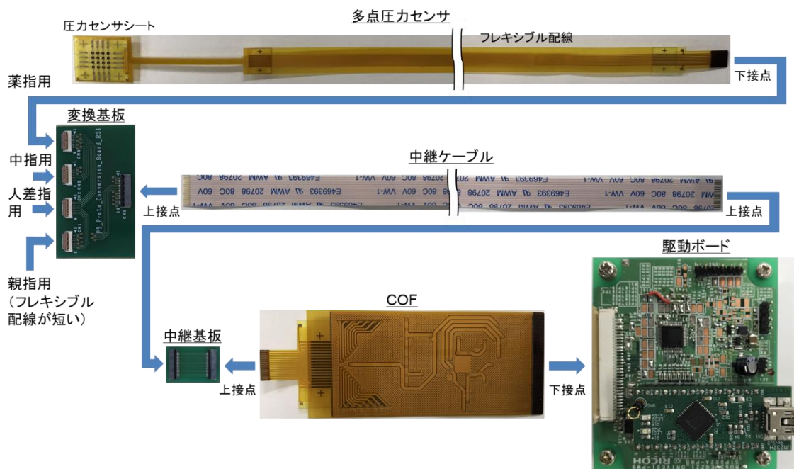
図 2 16 点センサ X4 セットを用いた構成
