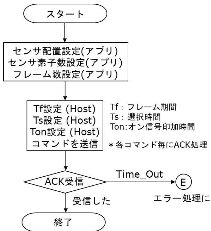
図 6 ボード設定処理フロー
