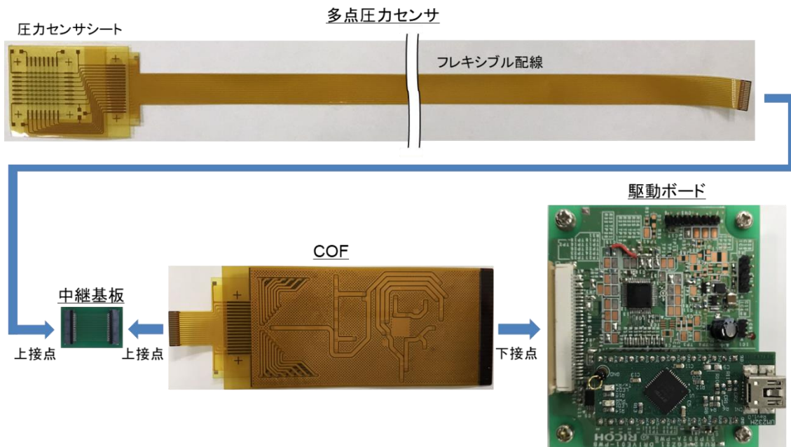
図1 64点センサを用いた構成
