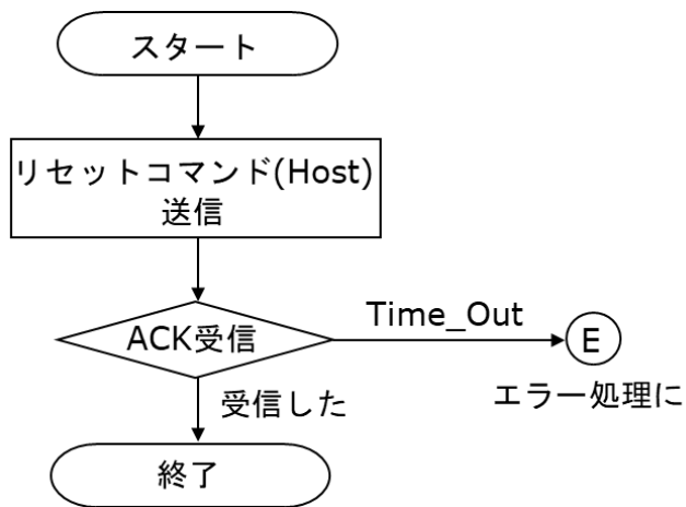
図 5 リセット処理フロー
