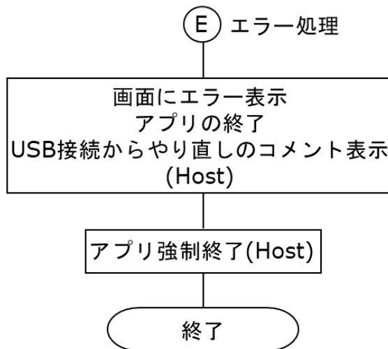
図11 エラー処理フロー
